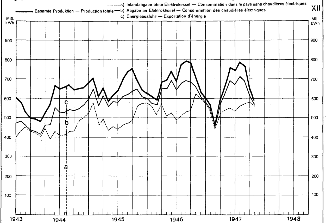
Energieproduktion der Elektrizitätswerke der allgemeinen Versorgung — Production d'énergie des usines électriques publiques
